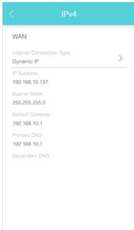
IPv4
