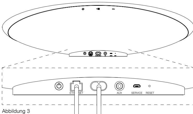
Abbildung 3 Setup bei einer kabelgebundenen Verbindung
