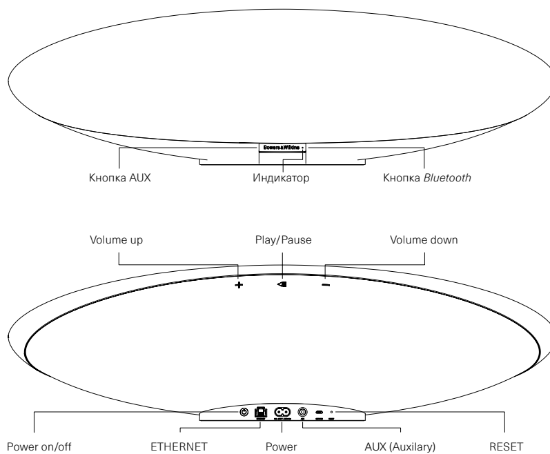
Рисунок 1 Кнопки и разъемы для подключения
